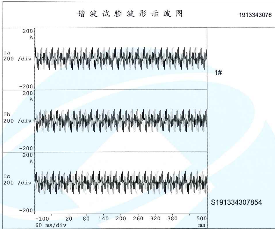
谐波测试示波图
