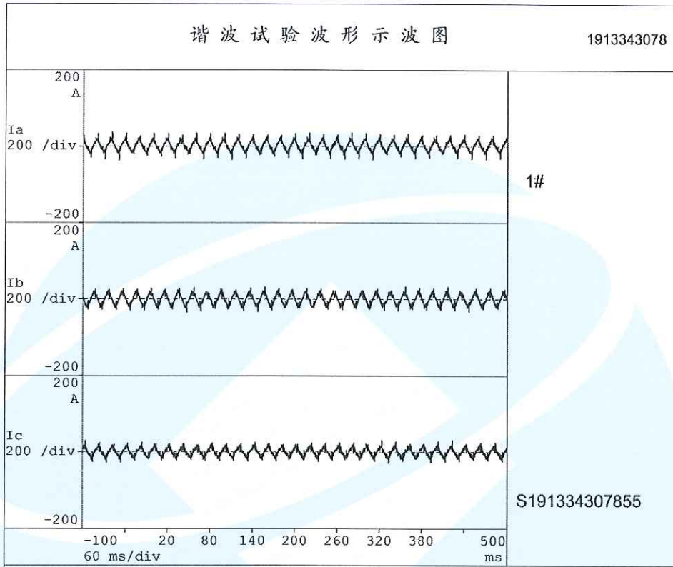
谐波测试示波图
