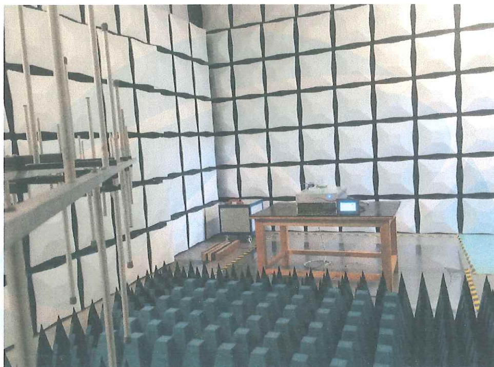
辐射电磁场干扰试验布置图:
