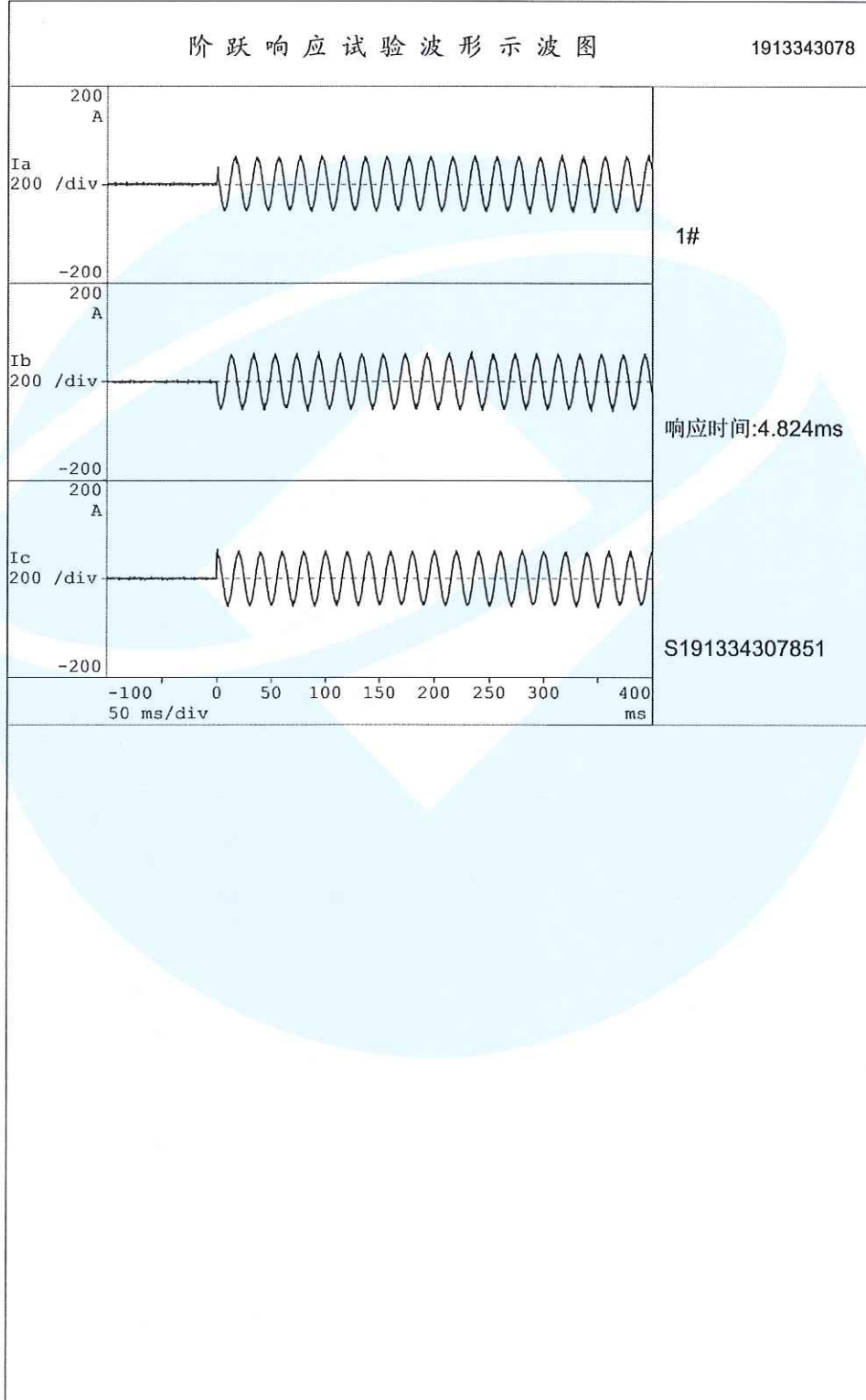
阶跃响应试验示波图
