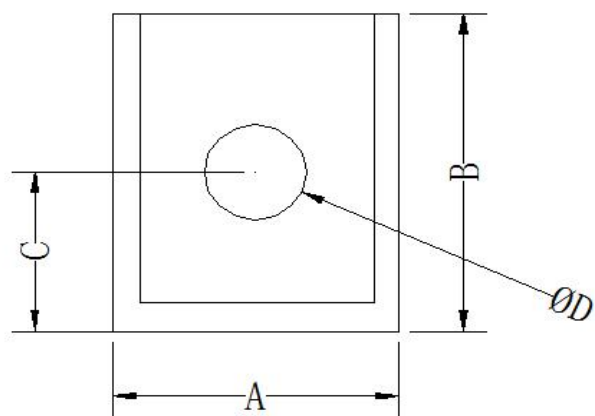
端子尺寸图
